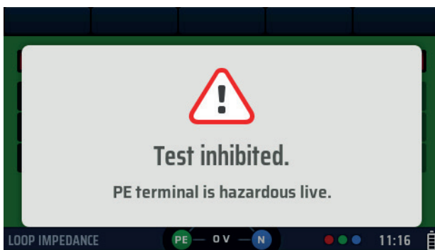
Afb.33: Blokkering PE-waarschuwing
