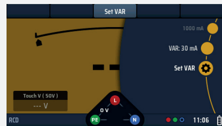
Afb.50: Set VAR-optie
