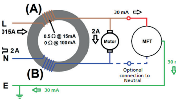
Afb.46: Vereenvoudigd aardlekschakelaarcircuit
