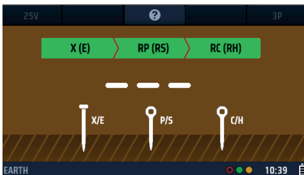
Afb.27: 3P aarde
