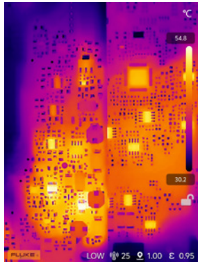
Printplaten
