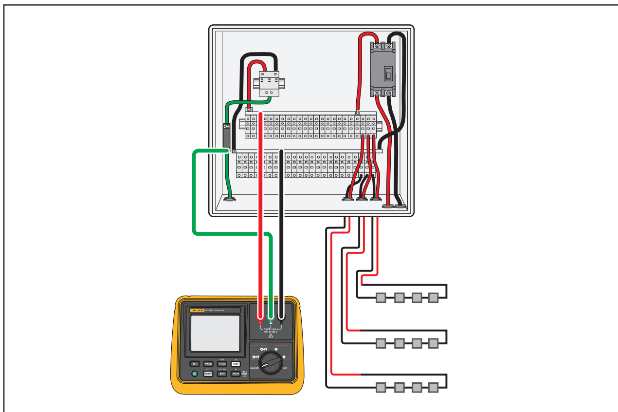
Afbeelding 13. Dubbel gezeekerde aansluiting van de combinerbox
