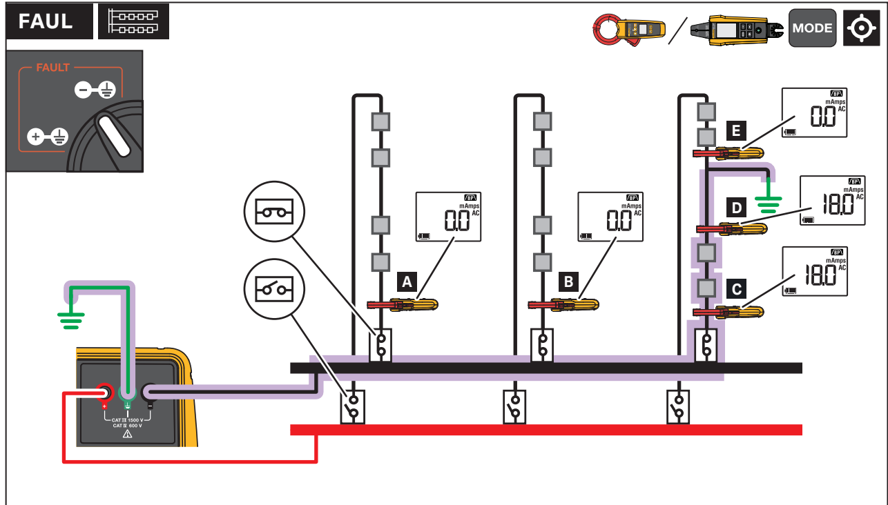
Afbeelding 14. Een fout met onderbroken zekeringen lokaliseren
