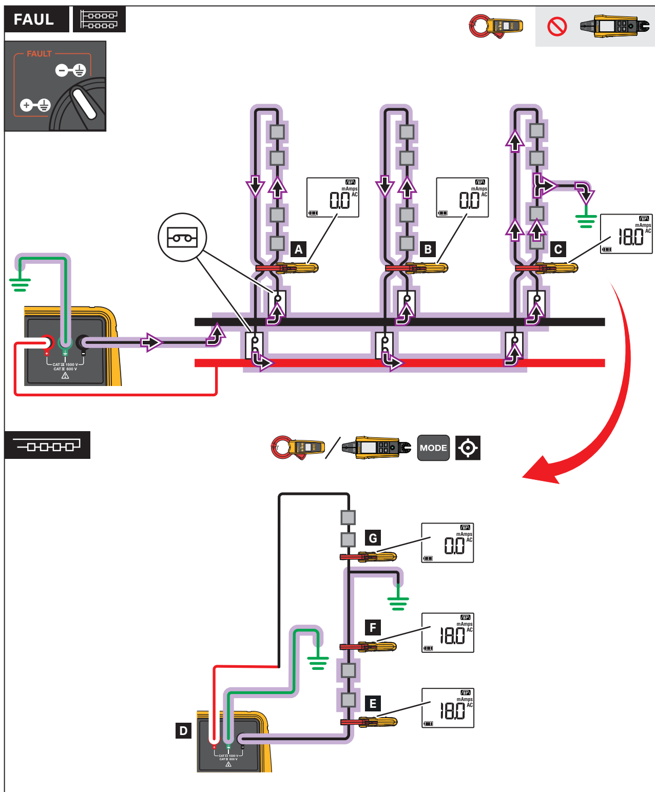
Afbeelding 16. Een fout met gesloten zekeringen lokaliseren
