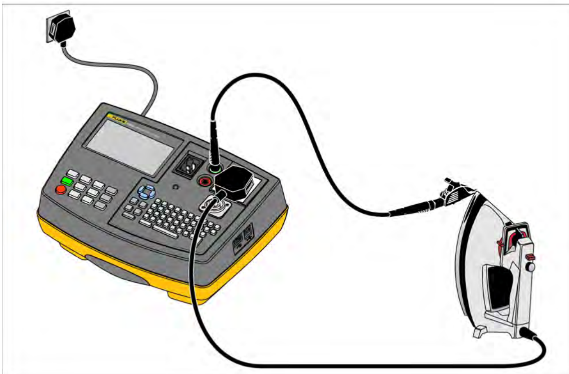
Afbeelding 2. Beschermingsleidingtest
