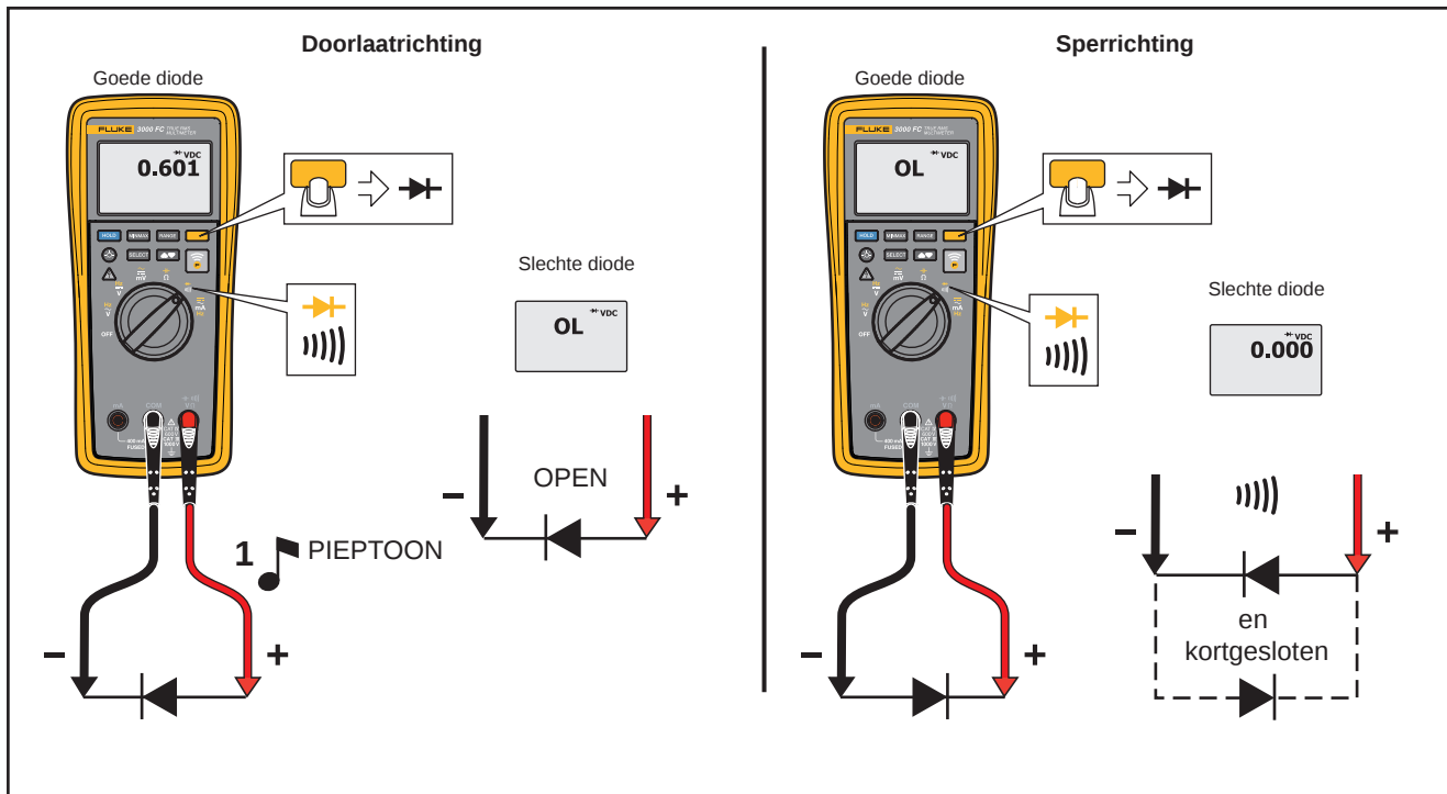
Afbeelding 7. Diodetest
