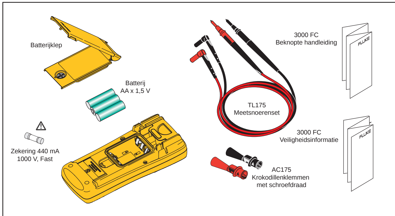
Afbeelding 11. Vervangende onderdelen
