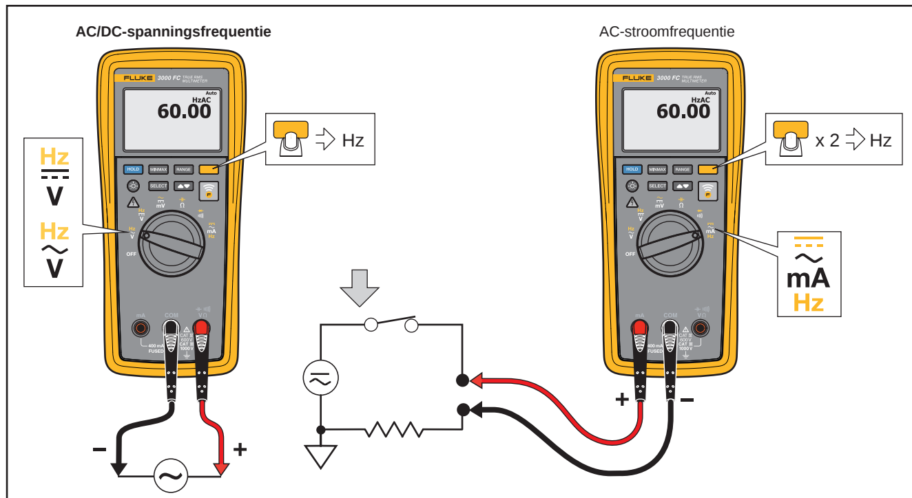
Afbeelding 8. Frequentiemeting
