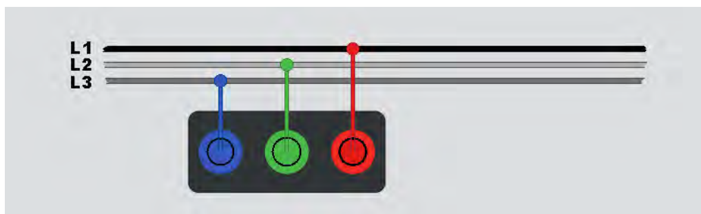
Afbeelding 20. Aansluiting voor faserotatietest
