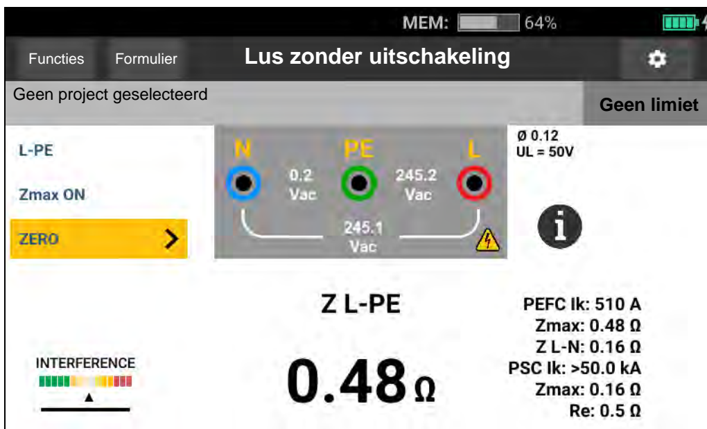
Afbeelding 11. Scherm Lusimpedantiemeting zonder uitschakeling
