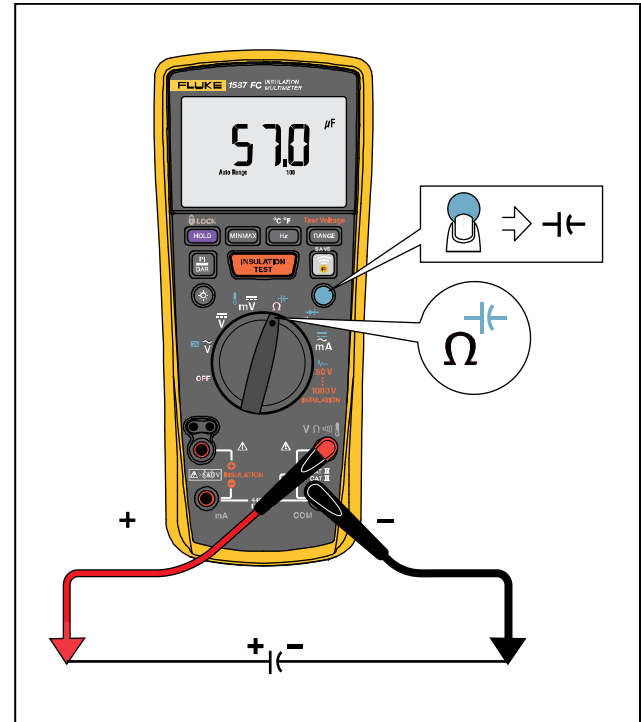
Afbeelding 5. Capaciteit meten
