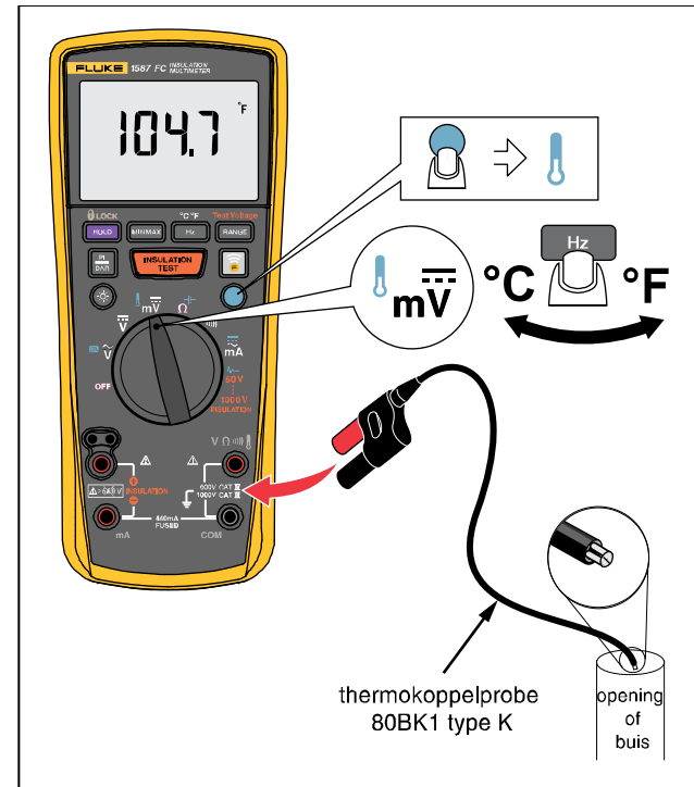
Afbeelding 3. Temperatuur meten
