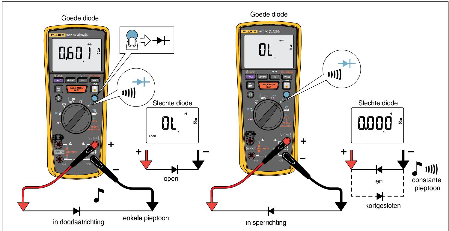
Afbeelding 7. Diodes testen
